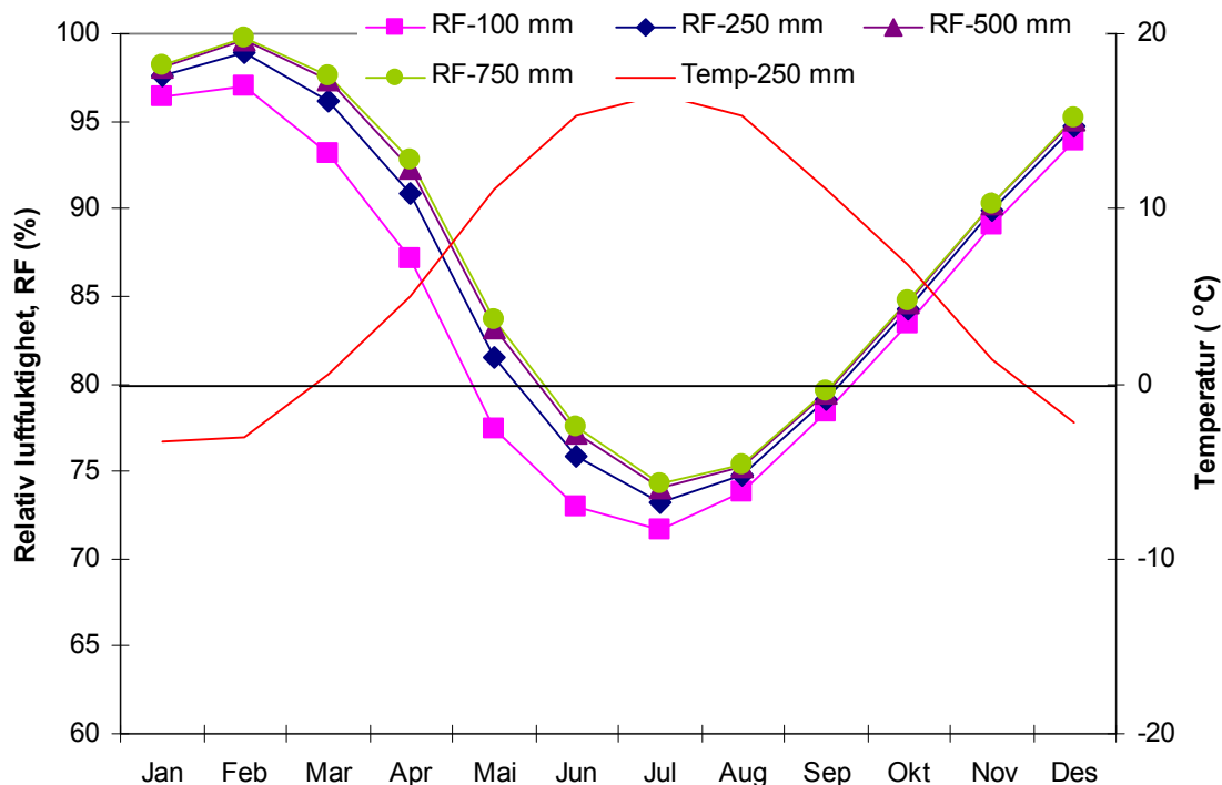
Figur 4.5 RF og temperatur på innsiden av undertaket på det kalde luftede loftet for forskjellige isolasjonstykkelser i himlingen. Sted = Oslo. Husets lekkasjetall = 4,0 \text{ m}^3/\text{m}^3\text{h}50\text{Pa} . Spalteåpning v/raft = 1 mm (dvs. redusert ventilasjon av loftet) . Fuktproduksjon = 10 \text{ kg/døgn} . Når RF og temperatur samtidig er over hhv 80% og 0^\circ\text{C} (over den heltrukne linjen) er det risiko for muggvekst.
