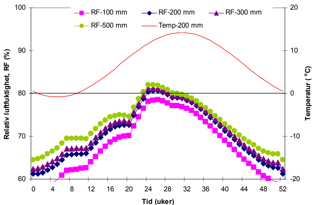
Figur 5.4 RF og temperatur midt i kryperommet for forskjellige isolasjonstykkelser i kryperomshimlingen. Referansetilfelle: Sted = Oslo. Kryperomnets luftskifte = 2,0 1/h. Ingen ekstra varmeisolasjon på grunnen. 0,2 mm plastfolie på grunnen. Beregningsperiode 1. januar – 31. desember. Når RF og temperatur samtidig er over hhv 80% og 0 °C (over den heltrukne linjen) er det risiko for muggvekst.
