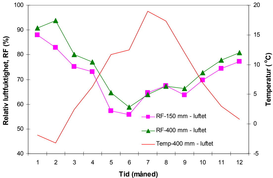
Figur V1.6 RF på vindsperras indre overflate for konstruksjon A, for hhv. 150 og 400 mm varmeisolasjon. Effekt av ventilert luftspalte. Luftspalten bak kledningen er modellert med et luftskifte på 20 1/h. Ellers er beregningsforutsetningene de samme som for standardtilfellene nr 1 og nr 3: Beregningsperiode 1. januar – 31. desember. S_d -dampsperre = 10 m. S_d -vindsperre = 0,23 m. Uteklime er Oslo. Fukttilskudd = 4 \text{ g/m}^3 . Månedsmiddelverdier.
