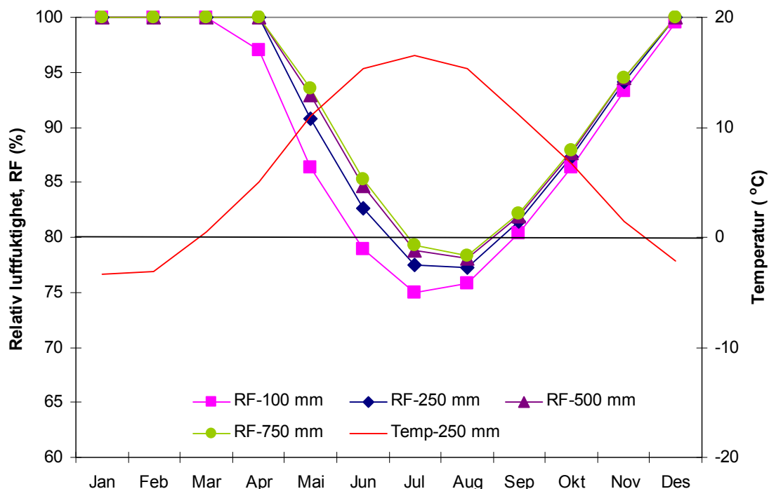
Figur 4.6 RF og temperatur på innsiden av undertaket på det kalde luftede loftet for forskjellige isolasjonstykkelser i himlingen. Sted = Oslo. Husets lekkasjetall = 4,0 \text{ m}^3/\text{m}^3\text{h}50\text{Pa} . Spalteåpning v/raft = 1 mm. Fuktproduksjon = 15 \text{ kg/døgn} (dvs. både redusert ventilasjon av loftet og høyere fuktinnhold i den lufta som lekker opp på loftet) . Når RF og temperatur samtidig er over hhv 80% og 0^\circ\text{C} (over den heltrukne linjen) er det risiko for muggvekst.
